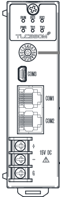
메인유닛(TLC990ME)의 정면
